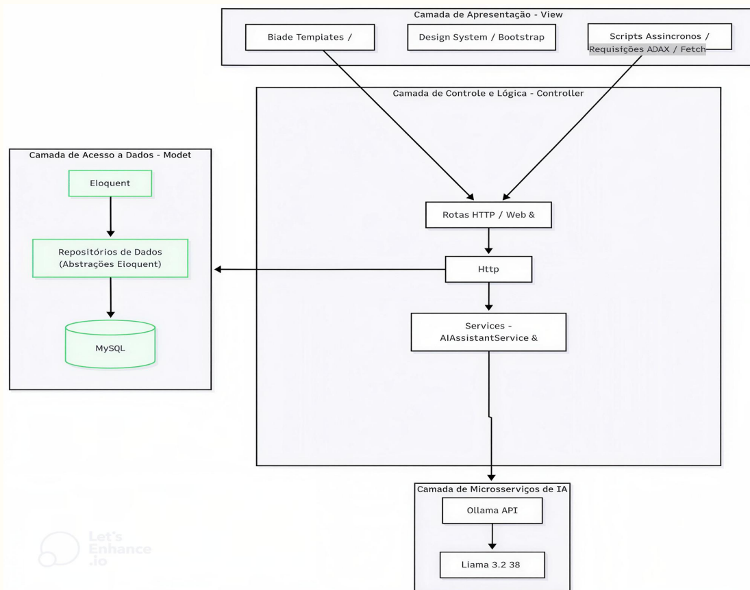
Figura 2 - Diagrama de Pacotes e Camadas de Dependências de Software.
